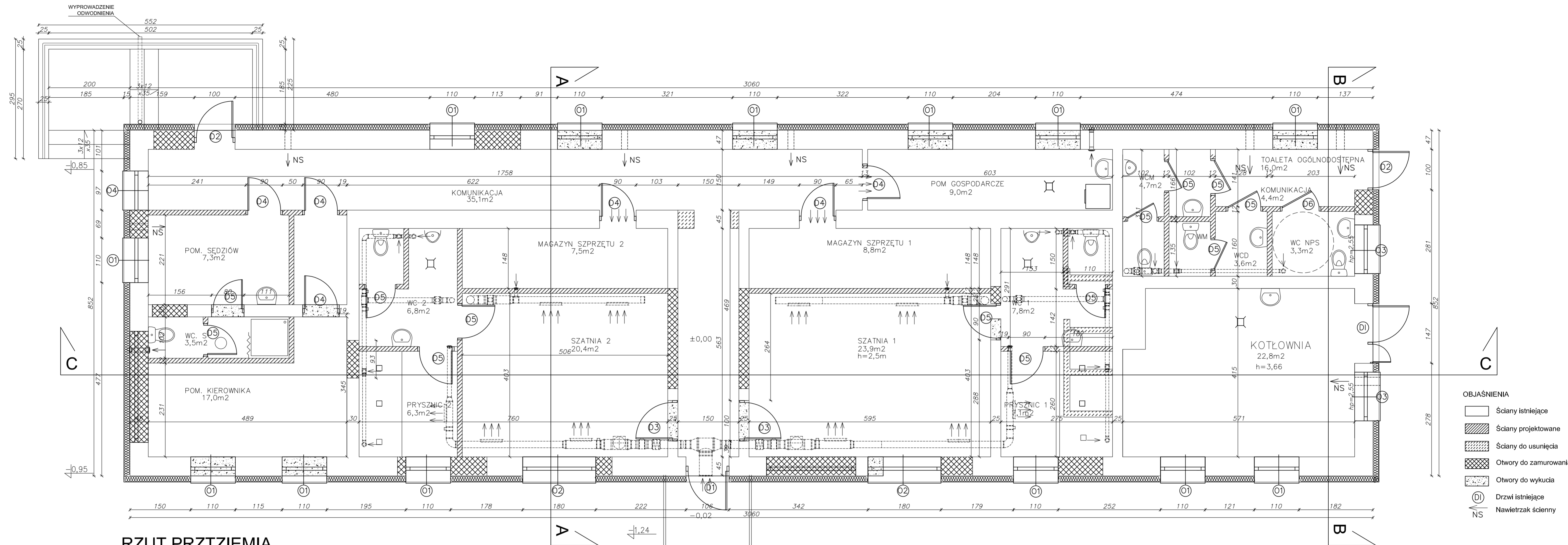
RZUT PRZTZIEMIA
